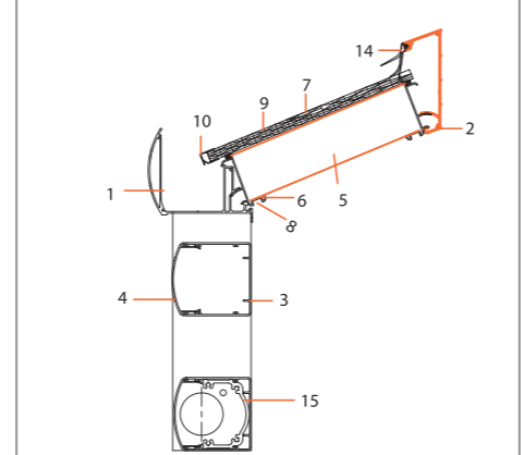
PROFİL DETAY
