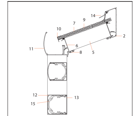
PROFİL DETAY
